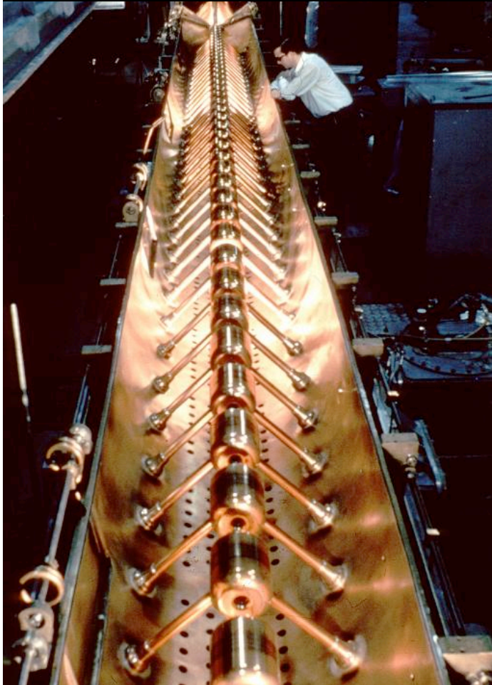
LINAC 1 (CERN)
